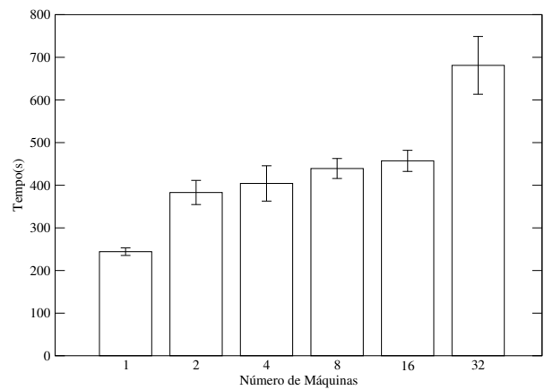
Figura 4. Tempo total de implantação do Inte-Grade em um aglomerado de máquinas
