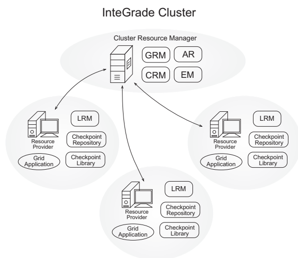
Figura 2. Arquitetura de um aglomerado InteGrade
