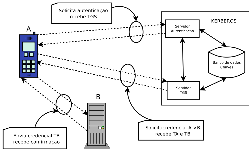
Figura 2.7. Protocolo do Kerberos.
