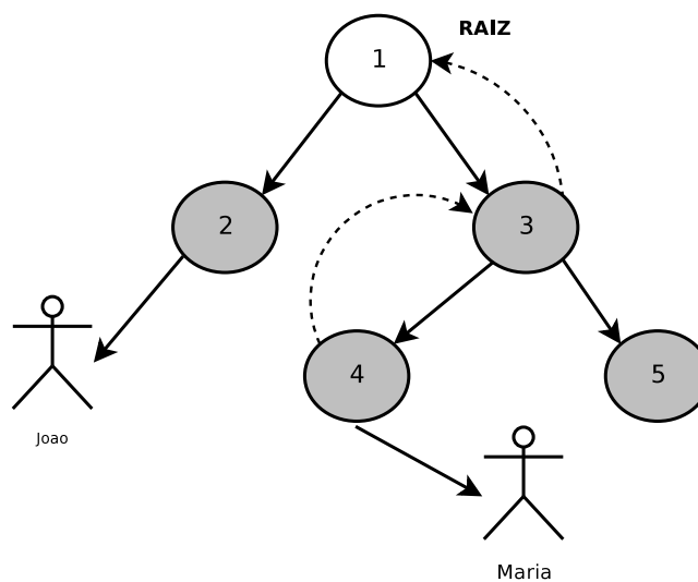
Figura 2.9. Hierarquia de Autoridade Certificadora.
