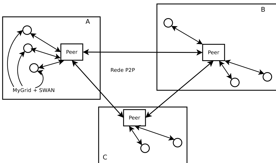
Figura 2.23. Arquitetura do OurGrid.
