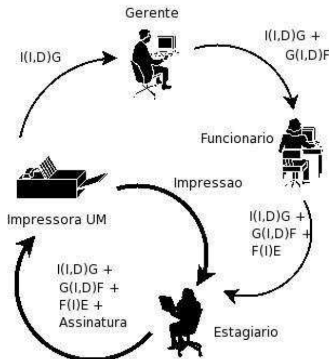
Figura 2.13. Delegação de um Certificado.
