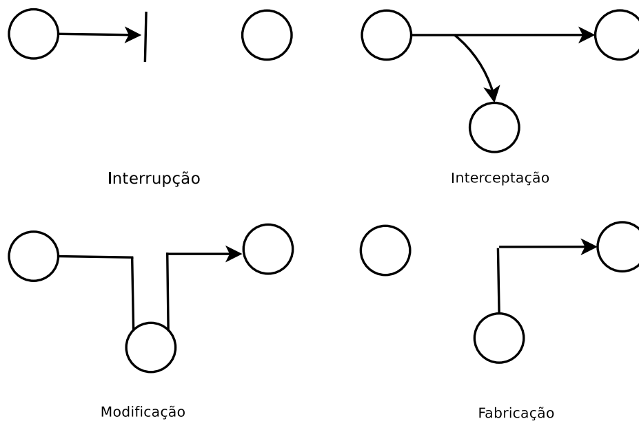
Figura 2.1. tipos de ataques [Stallings, 2002].
