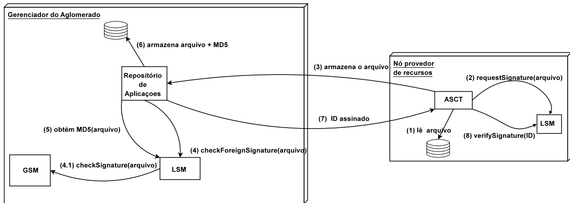
Figura 2.21. Protocolo de armazenamento de um executável de uma aplicação.
