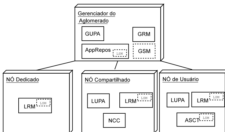
Figura 2.20. Arquitetura do InteGrade com os módulos de segurança.
