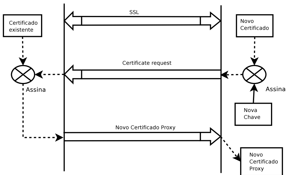
Figura 2.16. Delegação de Certificado Proxy
