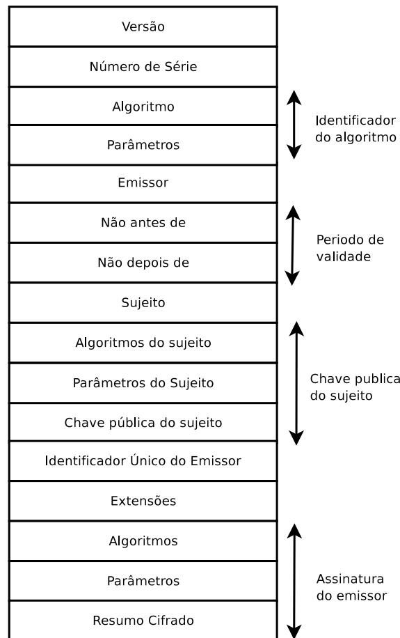
Figura 2.10. Campos que representam um Certificado de identidade X.509.
