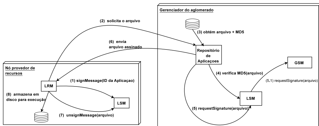
Figura 2.22. Protocolo de recuperação de um binário de uma aplicação.
