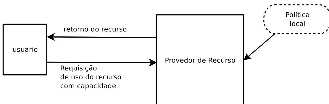
Figura 2.18. Cliente requisitando uso de recurso.
