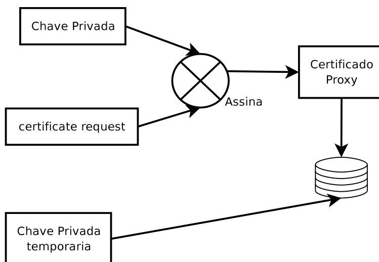
Figura 2.15. Protocolo de Autenticação Única.
