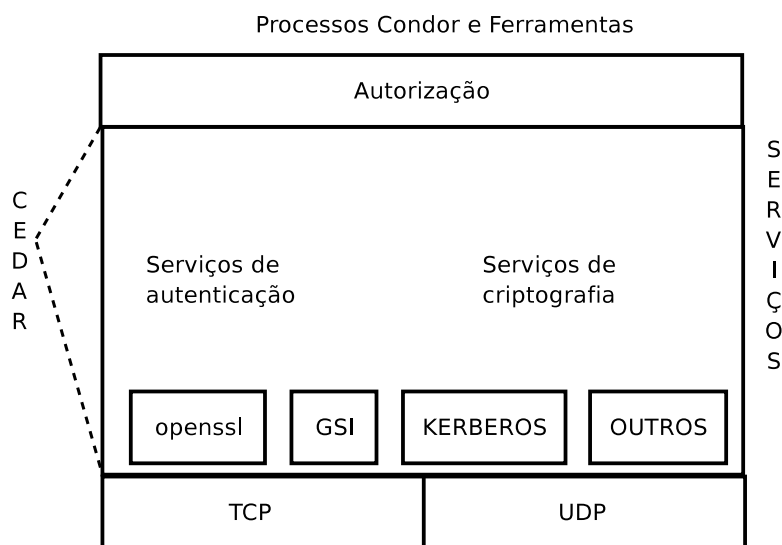
Figura 2.19. Arquitetura de Segurança do Condor.
