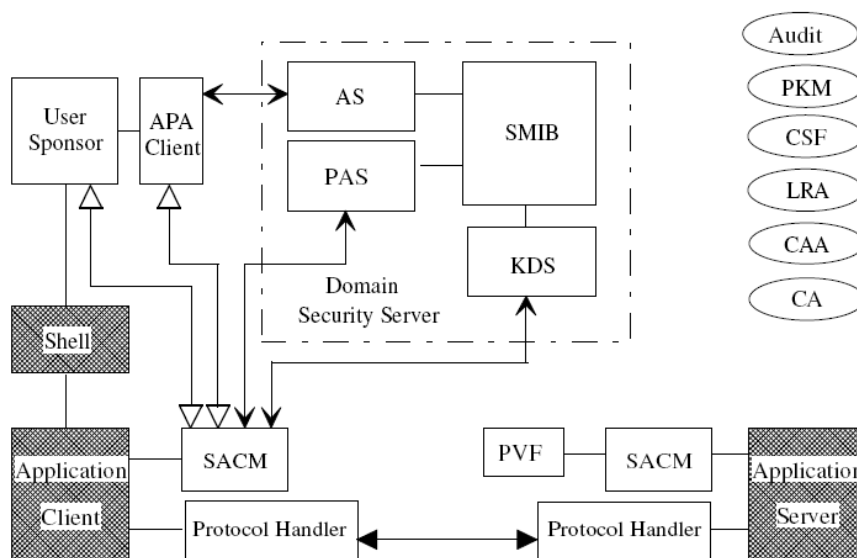
Figura 2.8. Arquitetura do SESAME [Sesame, 2003].
