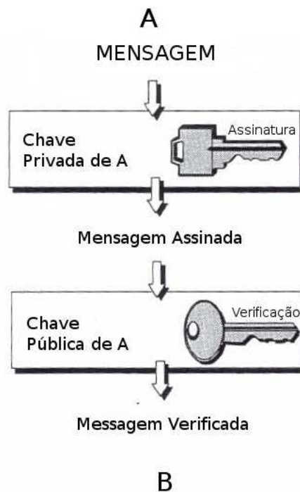
Figura 2.5. Assinatura através de uma chave pública.
