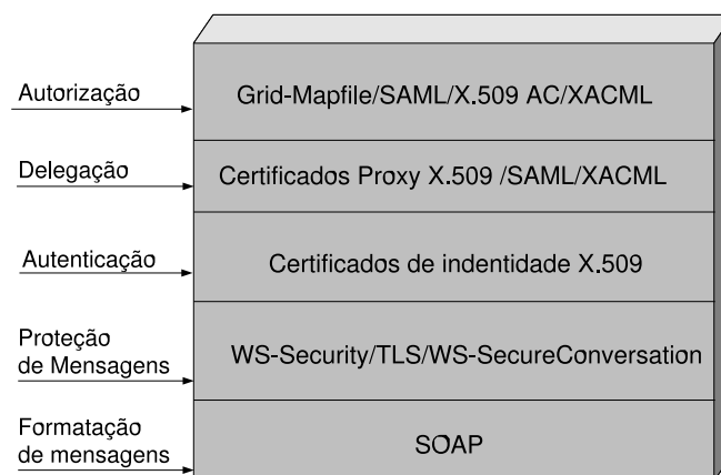
Figura 2.14. Arquitetura do GSI.
