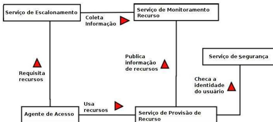
Figura 2.6. Arquitetura de uma Grade computacional.
