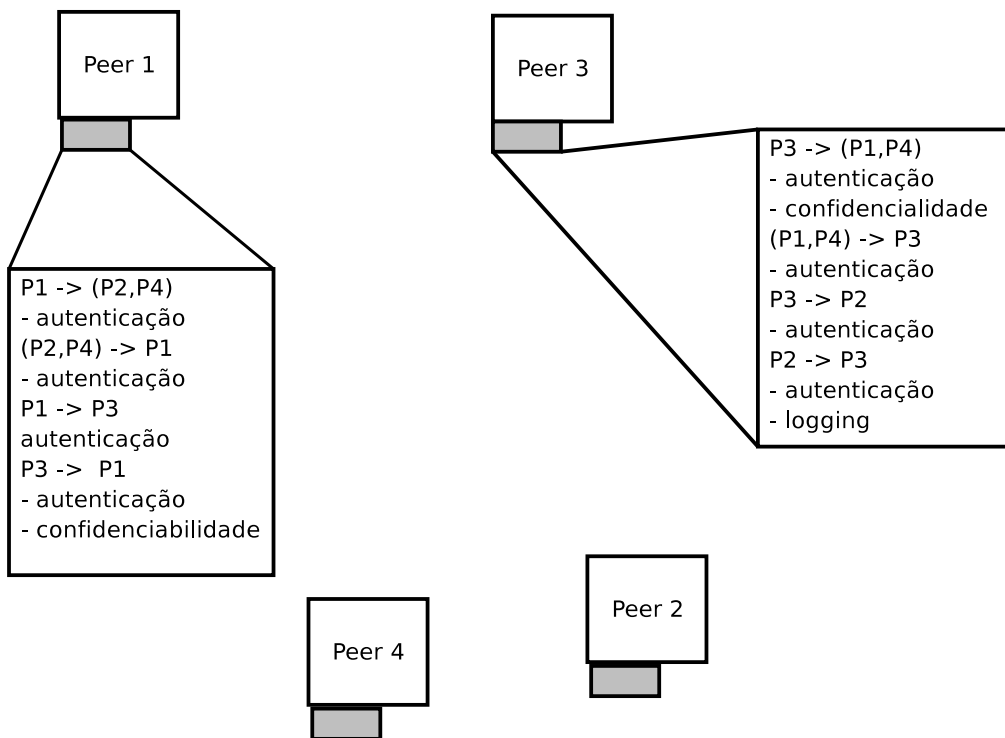
Figura 2.24. Arquitetura do P2PSFL.
